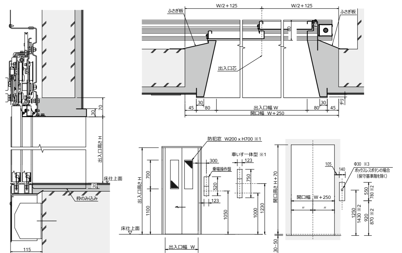
機種別出入口寸法一覧（ ）は有償付加仕様
