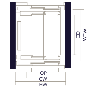
Ouverture latérale télescopique 2 faces de service
