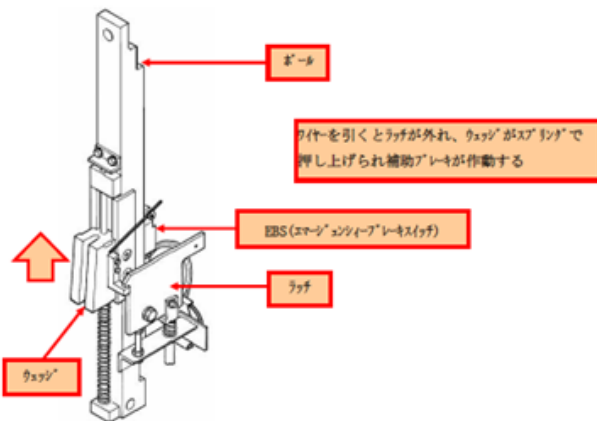
【ラッチがギヤより外側にある場合】
