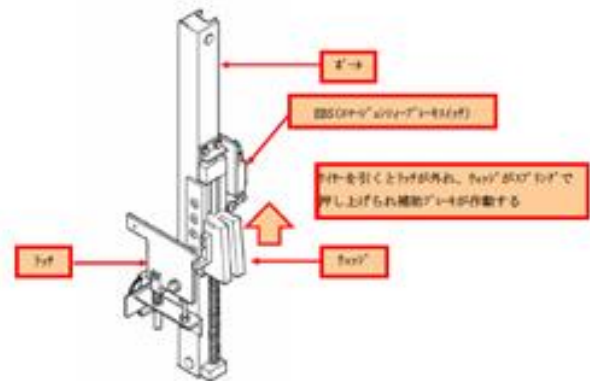
【ラッチがギヤより内側にある場合】
