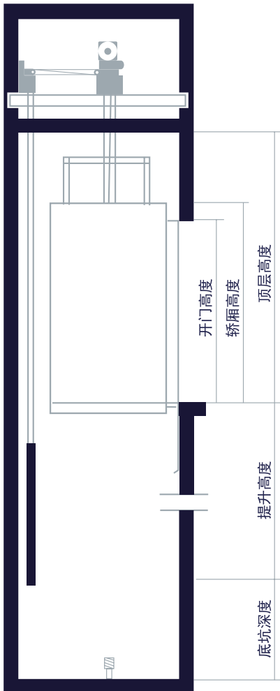
井道立面图
