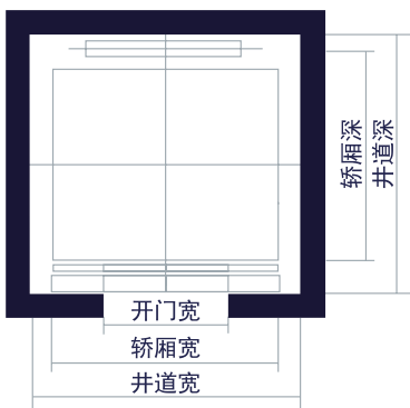
井道平面图
